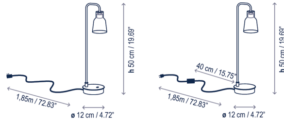
Interrupor Proxy Dimmer / Proxy Dimmer Switch Interrupor en el cable / Through cord switch
